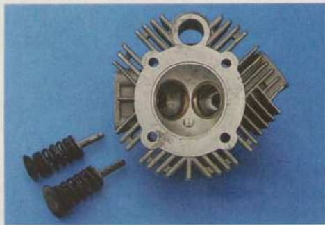
Problemfall: Manche Zylinderköpfe sind zu weich, gebrauchten Ersatz gibt's ab 250 Euro
