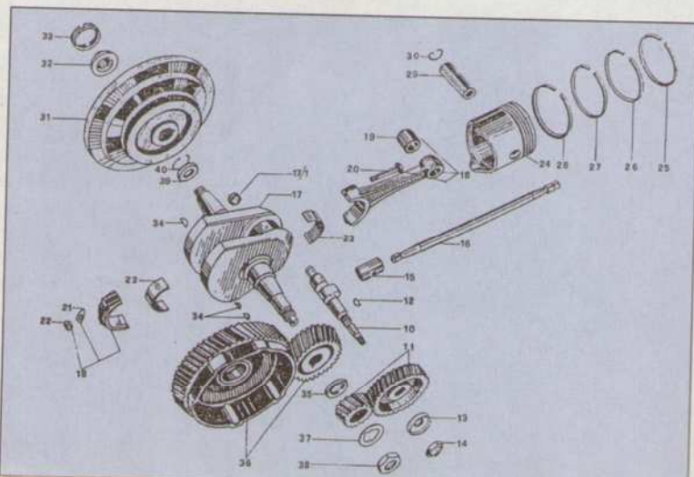
Erzsolide: der Kurbeltrieb. Laufleistungen von 100.000 Kilometern sind überliefert!
